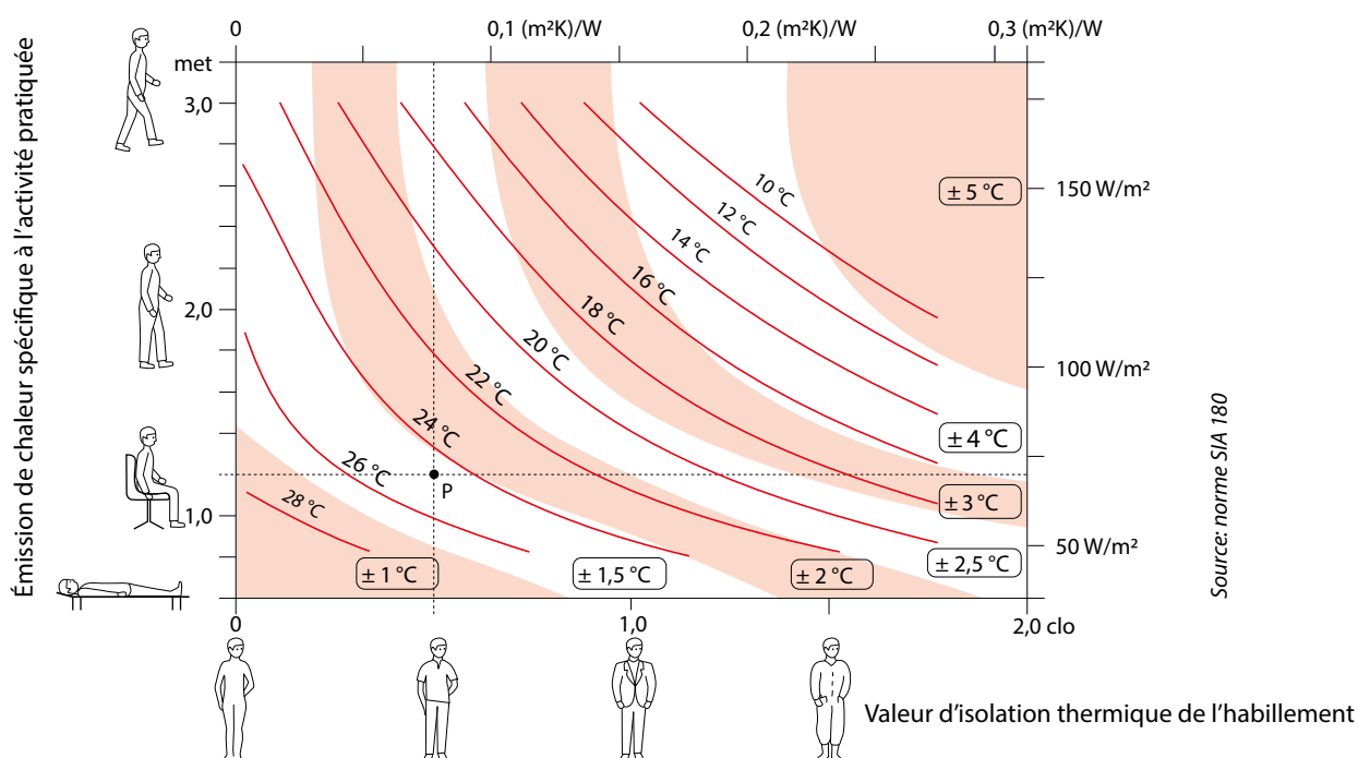
Fig. 3: températures ambiantes optimales en fonction de l'activité et de l'habillement. Exemple de lecture (P): un travail de bureau facile effectué en position assise (émission de chaleur spécifique 70 W/m² ou 1,2 met) avec habillement estival (résistance thermique 0,0775 (m²K)/W ou 0,5 clo) donne une température ambiante optimale ressentie de 24,5 °C avec une marge de tolérance de +/- 1,5 °C.
