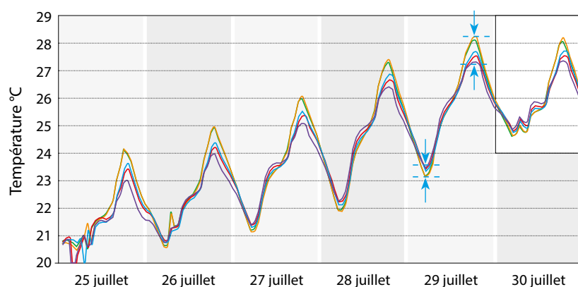
Fig. 10a: comme le montrent les courbes de température très proches, le choix du type d'isolant thermique est sans importance.
