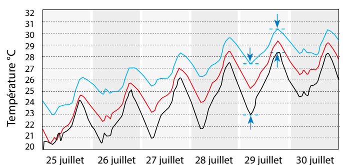
Fig. 9: comme le montrent les courbes de température noire et bleue (trois renouvellements d'air ou aucun), les différences de température peuvent atteindre 4,5 °C pendant la nuit et 2 °C pendant la journée (cf. flèches).
