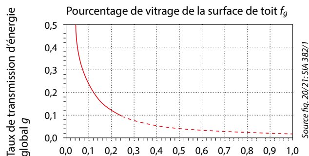
Fig. 17: exigences selon SIA 382/1 pour la valeur g des verrières (vitrage et protection solaire) en fonction du pourcentage de vitrage.
