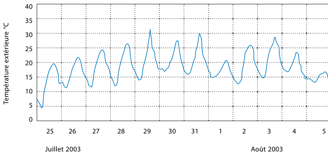
Fig. 6: courbe des températures extérieures Zurich-Kloten DRY juillet à août.
