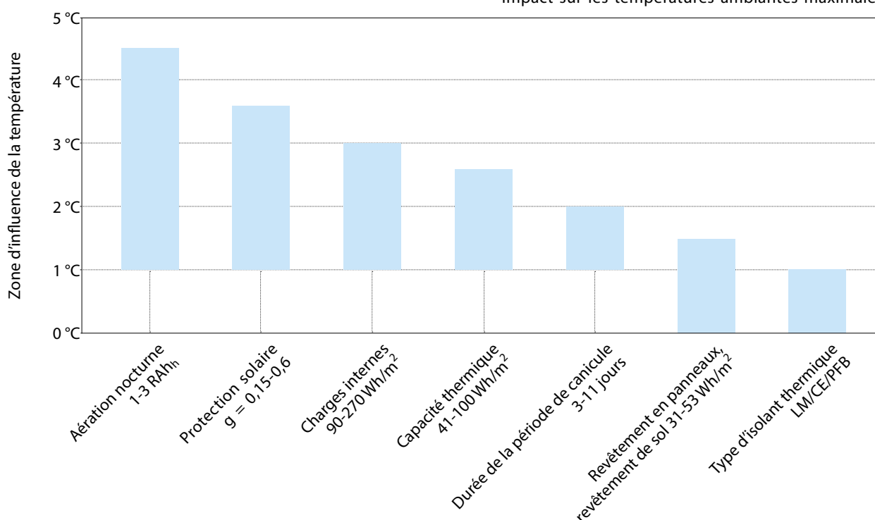
Fig. 12: montre clairement l'importance des différents facteurs d'influence. L'influence du type d'isolant thermique, de 0 à 1 °C max est insignifiante.
