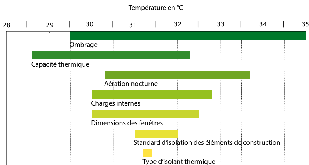
Fig. 14a: les différents facteurs et leur potentiel d'influence.
