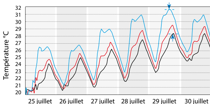
Fig. 8: même des dimensions de fenêtres modérées (20 % de la surface de sol; exposition est) entraînent des différences de température pouvant atteindre 3,5 °C. Les fenêtres plus grandes, exposées au sud ou les fenêtres de toiture entraînent des différences encore nettement plus importantes.
