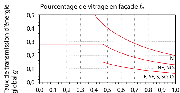
Fig. 16: exigences selon SIA 382/1 pour la valeur g des fenêtres en façade (vitrage et protection solaire) en fonction du pourcentage de vitrage et de l'orientation.
