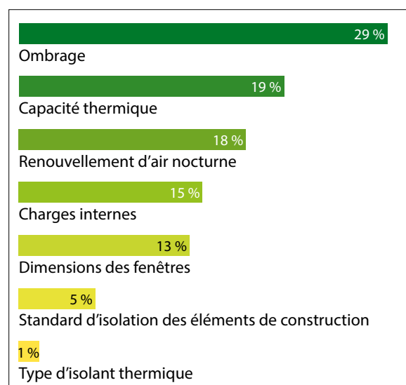
Fig. 14b: potentiel d'influence des différents facteurs en pourcentage.
