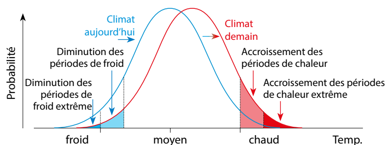
Fig. 2: accroissement des périodes de chaleur extrême, diminution des périodes de froid extrême
