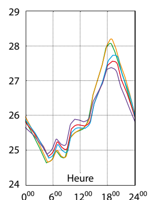
Fig. 10b: l'extrait agrandi montre les courbes de température au cours des 24 heures de la journée du 30 juillet DRY.
